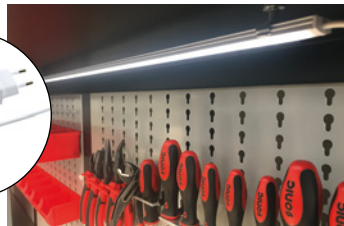
#4820524 MSS LED svetidlo so stmievačom - Dĺžka 600 mm - 400-500 lúmenov - Teplota farby: 6000-6500K
